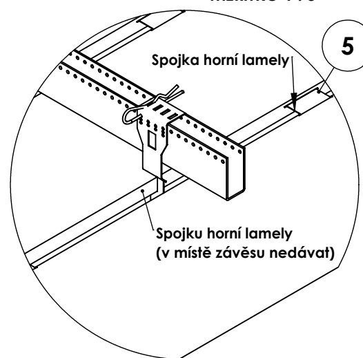
DETAIL E MĚŘITKO 1 : 5
