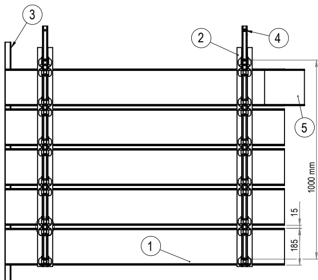
Podélný řez
